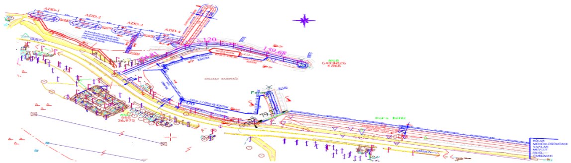
GÜLYALI BALIKÇI BARINAGI KAPASİTE ARTIRIMI ve KUM TUTUCU MENDİREK İNŞAATI İMAR PLANI ve ÇED ÇALIŞMALARI, ETÜT PROJE İŞLERİ ve FİZİBİLİTE ETÜDÜ GENEL VAZİYET PLANI Ö:1/5000
